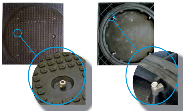
Détail point de levage
