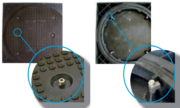
Détail verrouillage
