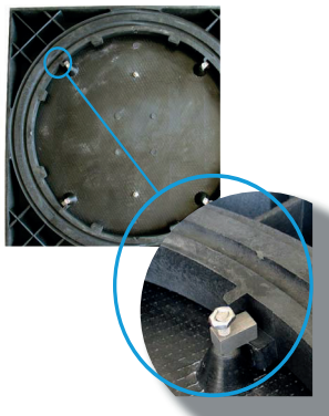
Détail verrouillage
